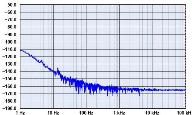
SLA36-7相位噪声测试曲线
