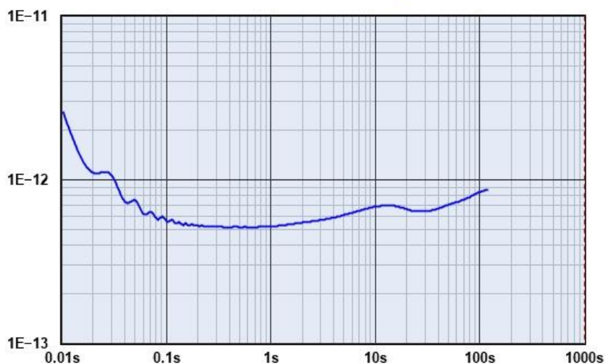
SLA36-10P阿伦方差
