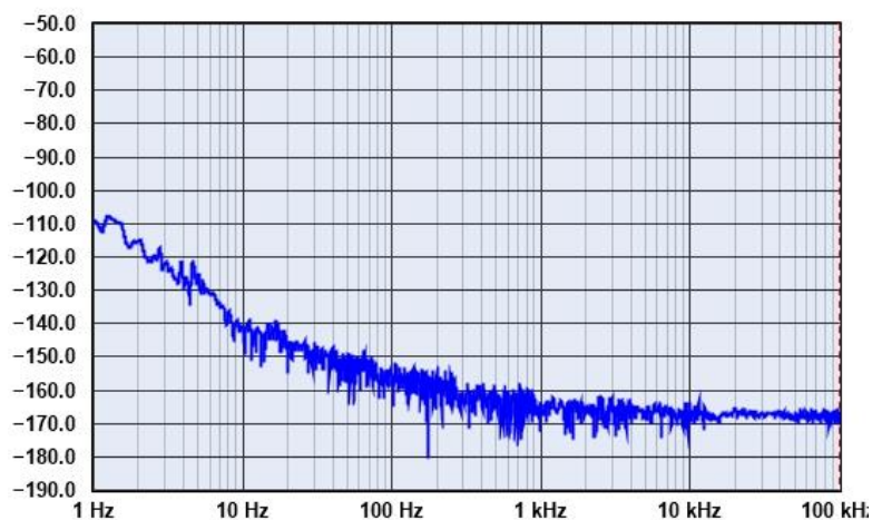
SLA36-10相位噪声测试曲线
