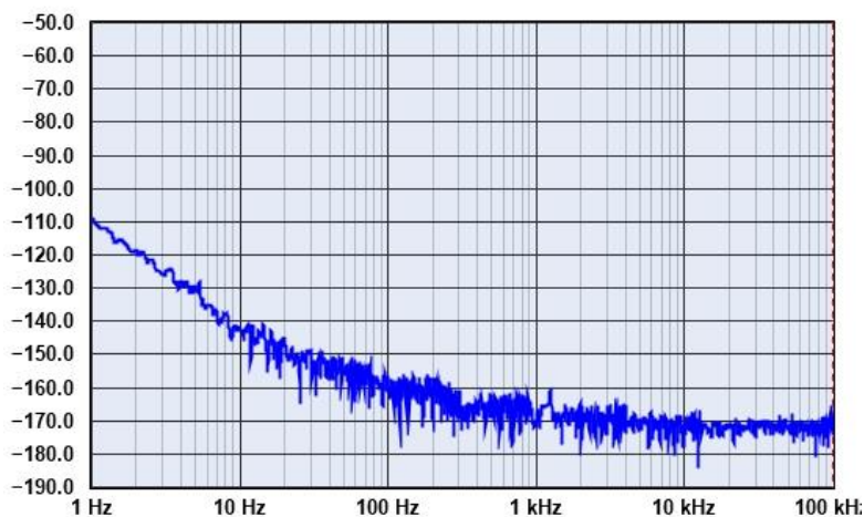
SLA36-10P相位噪声测试曲线
