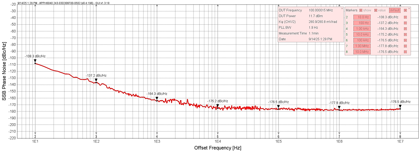
SLO12-155相位噪声测试曲线
