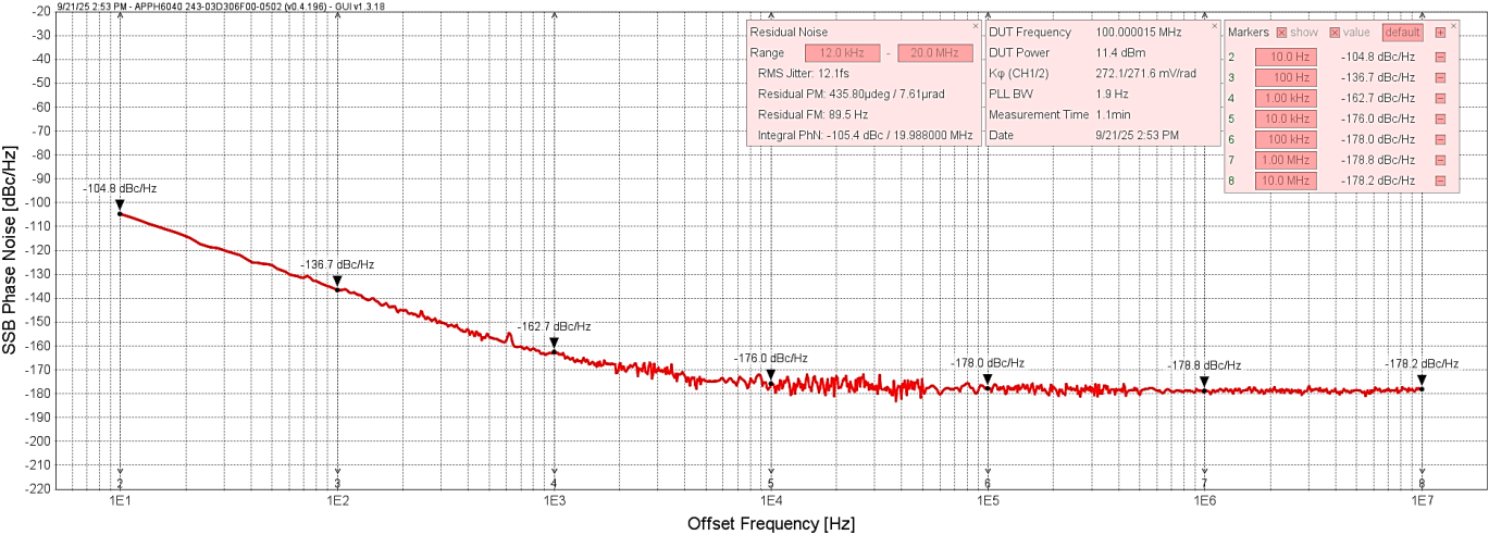
SLO20-160相位噪声测试曲线
