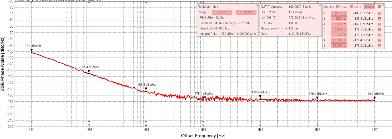
SLO25-160相位噪声测试曲线
