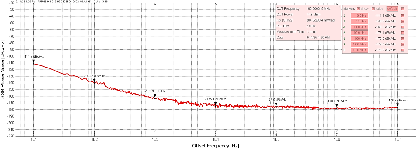
SLO12-160相位噪声测试曲线
