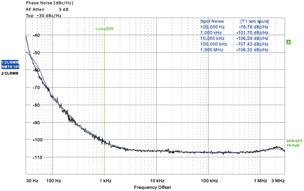
SWFA200在10GHz输出时相噪曲线
