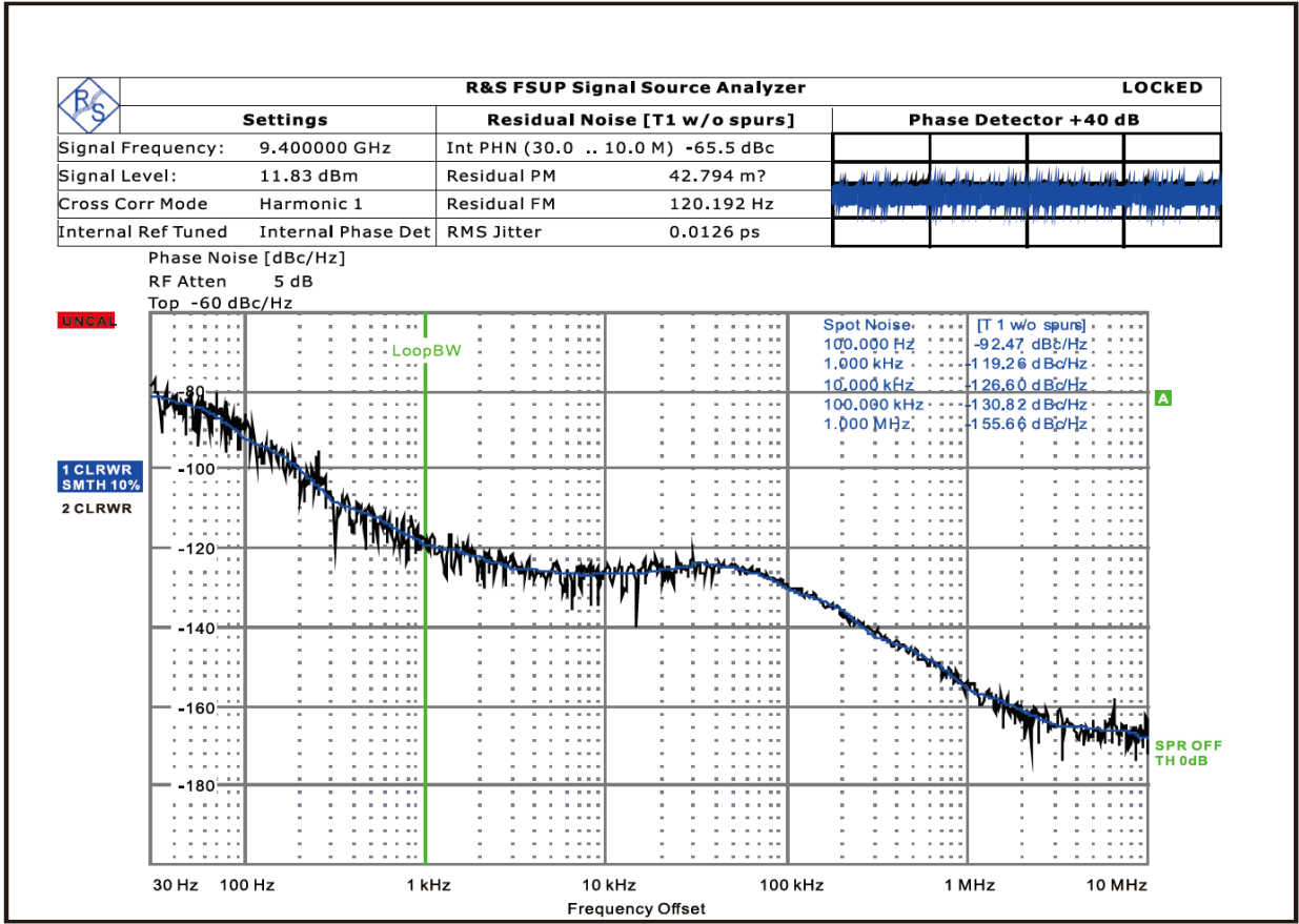
PDROxxxx系列9.4GHz输出时相位噪声
