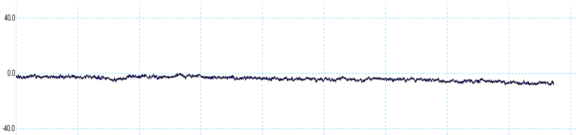
SMS1020 系列多通道间相位稳定度：9 小时小于 2°漂移
