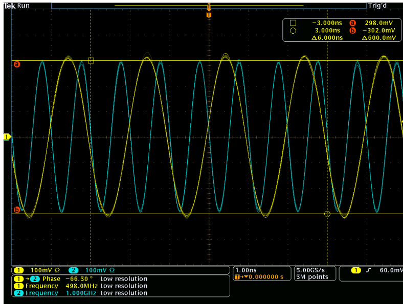
SMS1006 系列各通道频率、幅度、相位等独立可调
